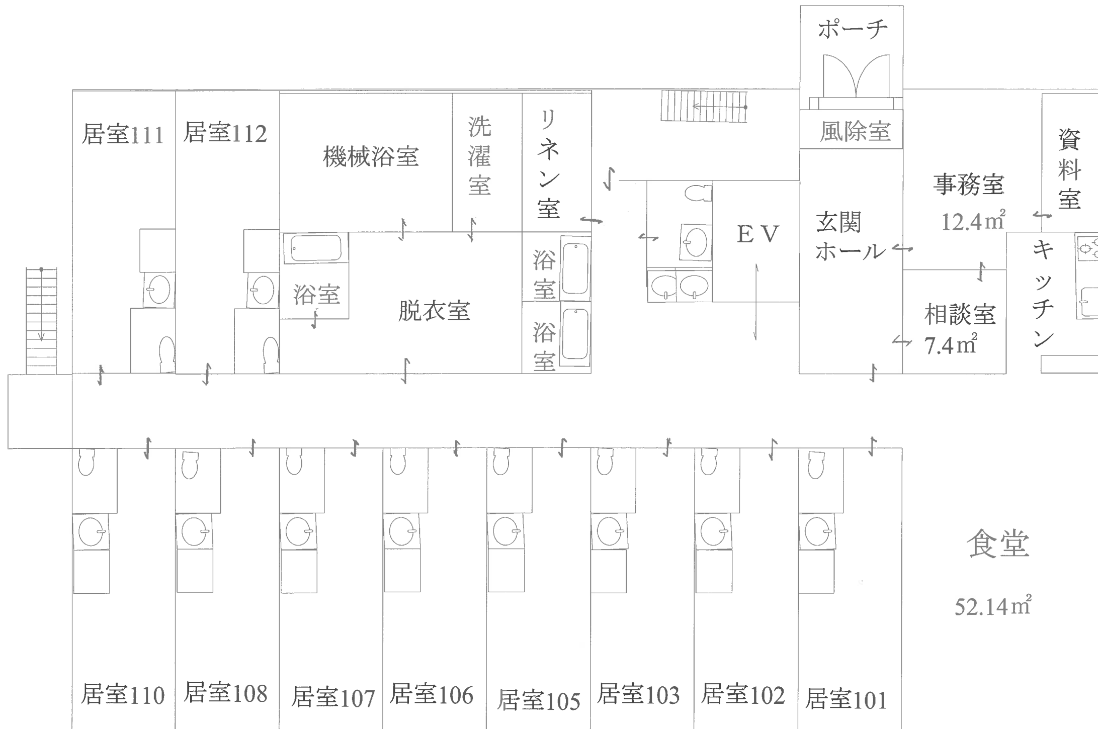
1階平面図 (各居室16.83m 2 )
